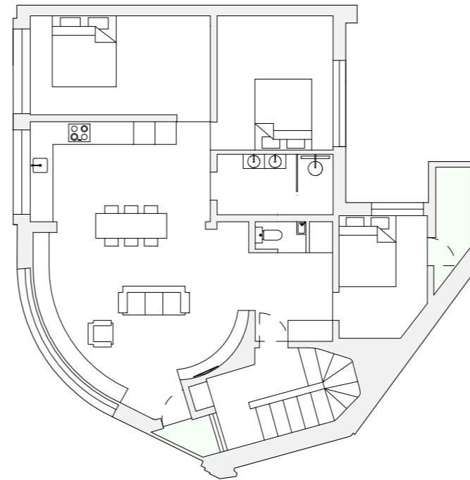
1° + 2° + 3° VERDIEPING
